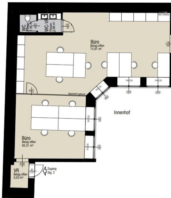
Grundriss M 1:100
