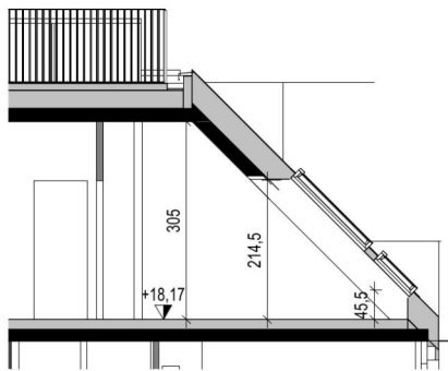
Schnitt 31.B
