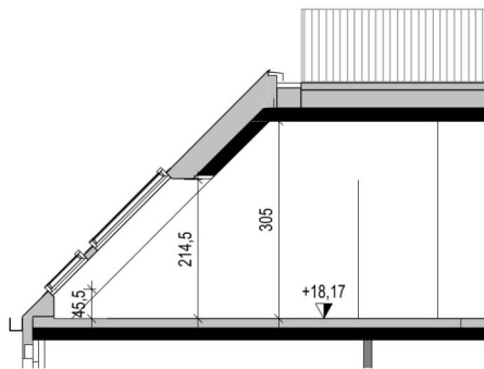
Schnitt 31.A
