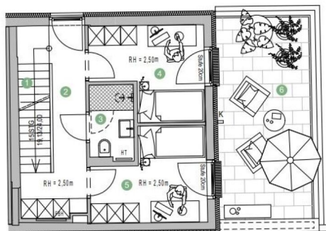
GRUNDRISS DG1
