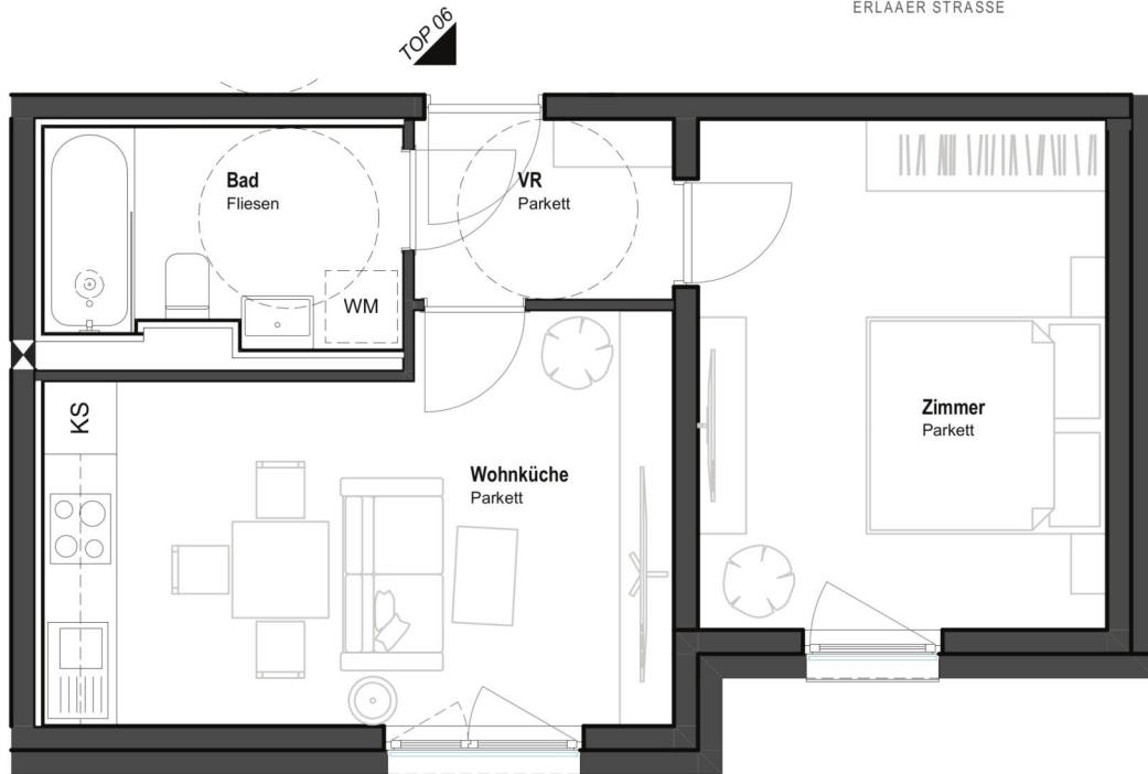
Grundriss 1:50
