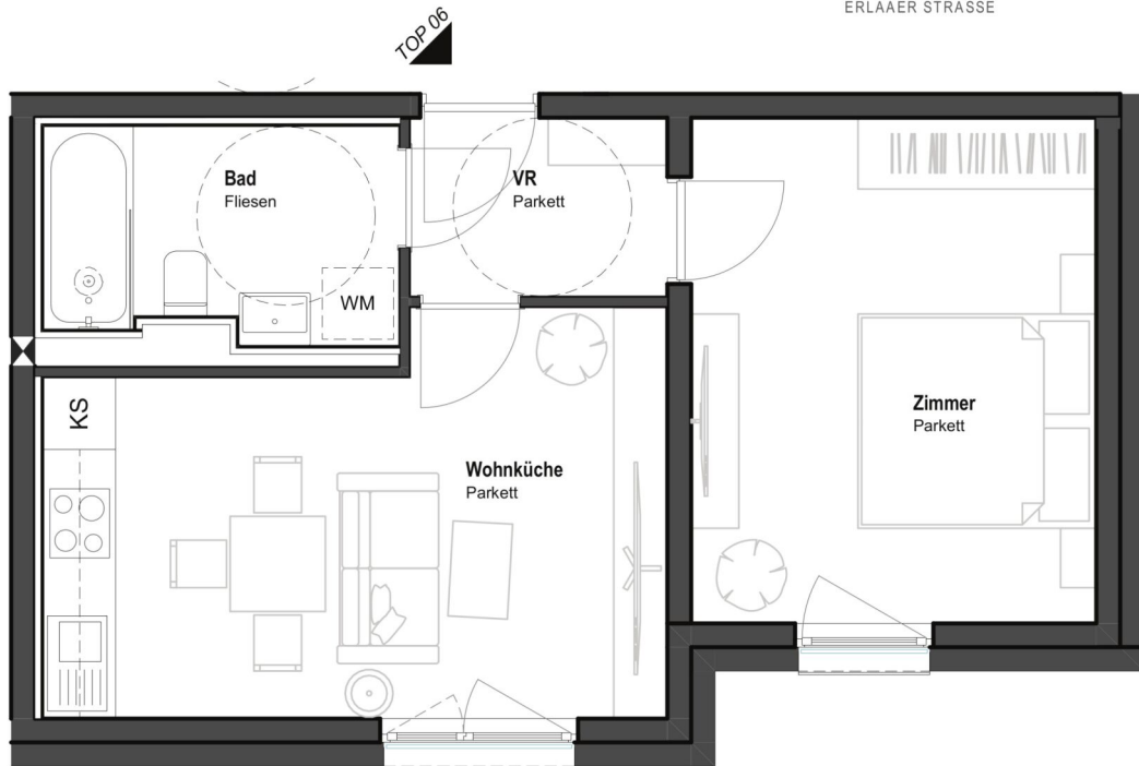
Grundriss 1:50
