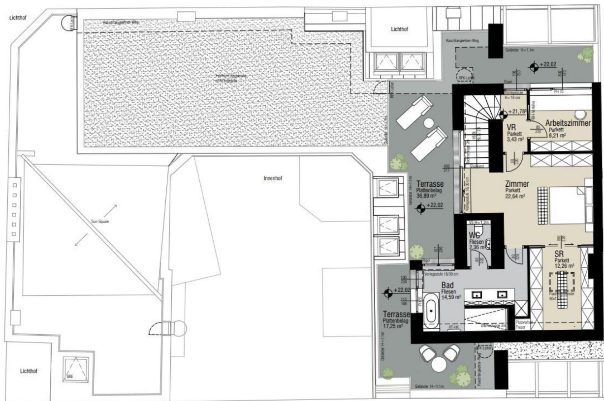
Grundriss M 1:100
