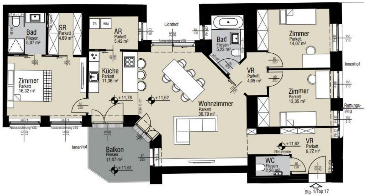
Grundriss M 1:100
