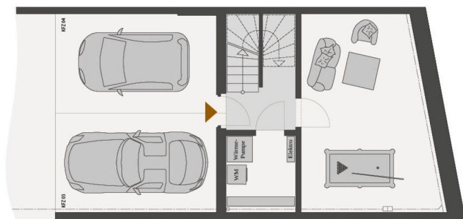
UNTERGESCHOSS
