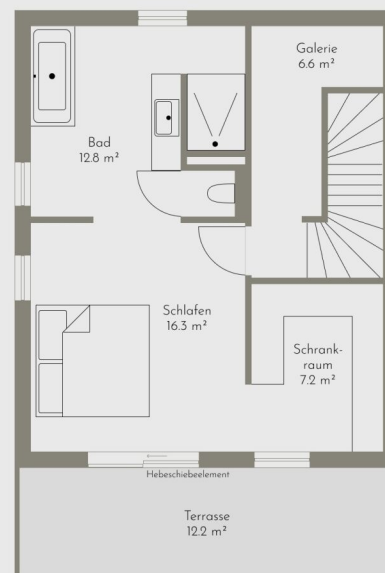
Dachgeschoss
