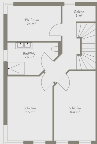
Obergeschoss
