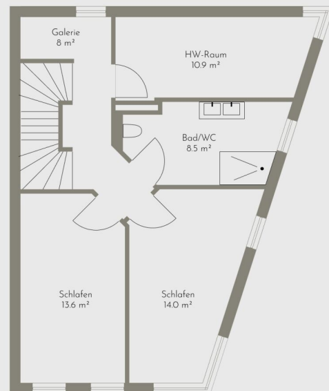
Obergeschoss
